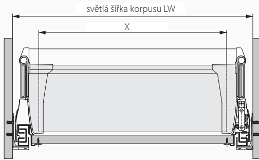
Optima profil pro Variowing X = LW - 96
